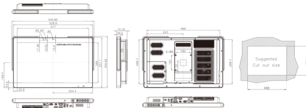
AFL2-W21-H61 Panel PC AFL2-W21-H61 Panel PC
