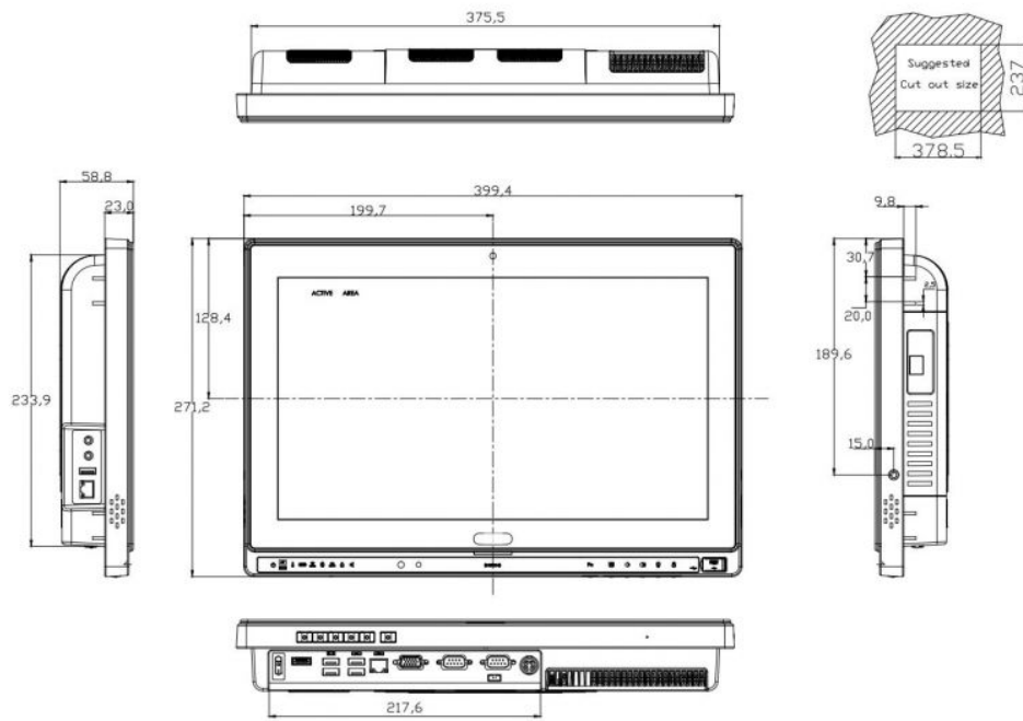
AFL2-W15B-H61 Panel PC Zeichnung
