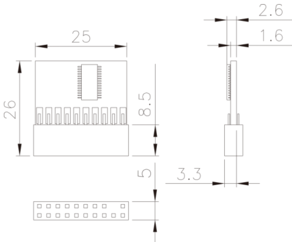
TPM-IN02-R20 Components Zeichnung
