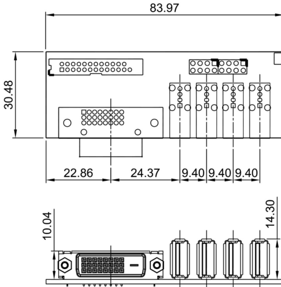
IO-KIT-001 Components bemaßte Zeichnung
