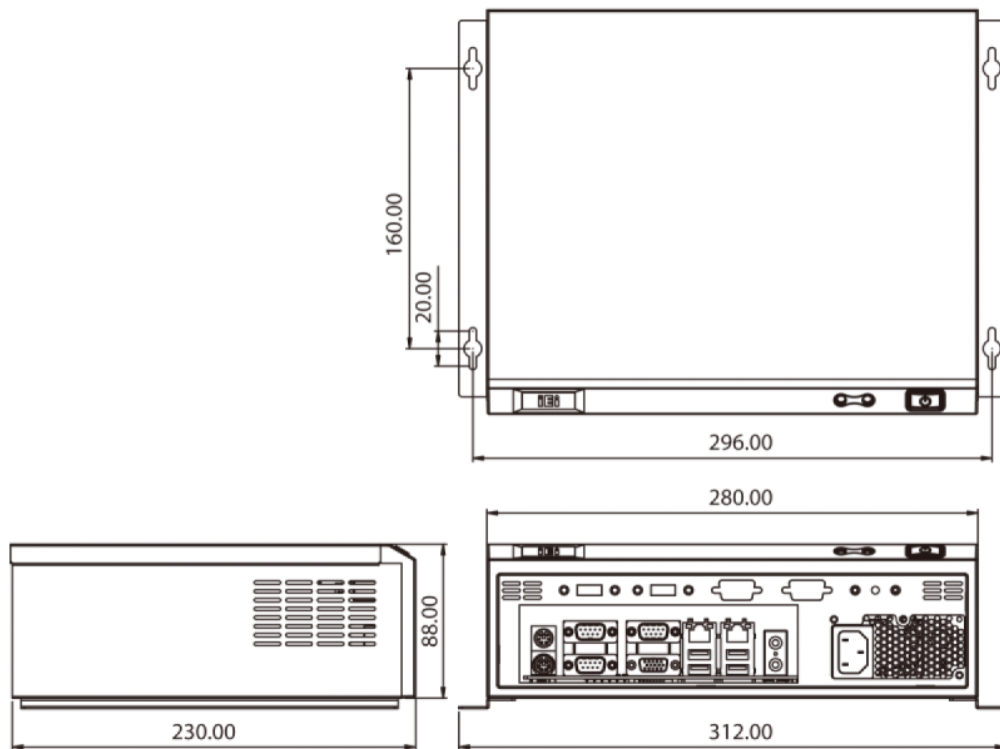
ebc-3000 Zeichnung bemaßte Normalprojektion
