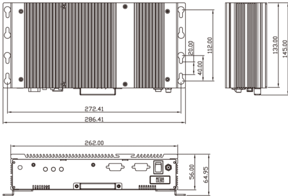
EBC-2100 bemaßte Zeichnung
