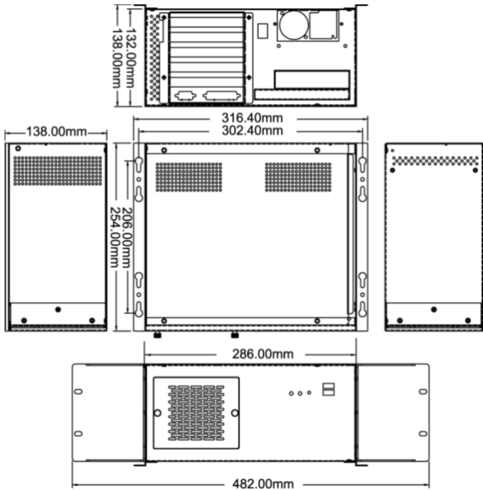
PR-1500G bemaßte Zeichnung
