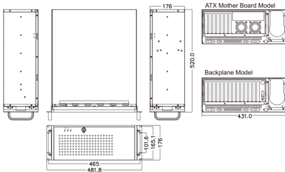
RACK-3000G Gehäuse bemaßte Zeichnung
