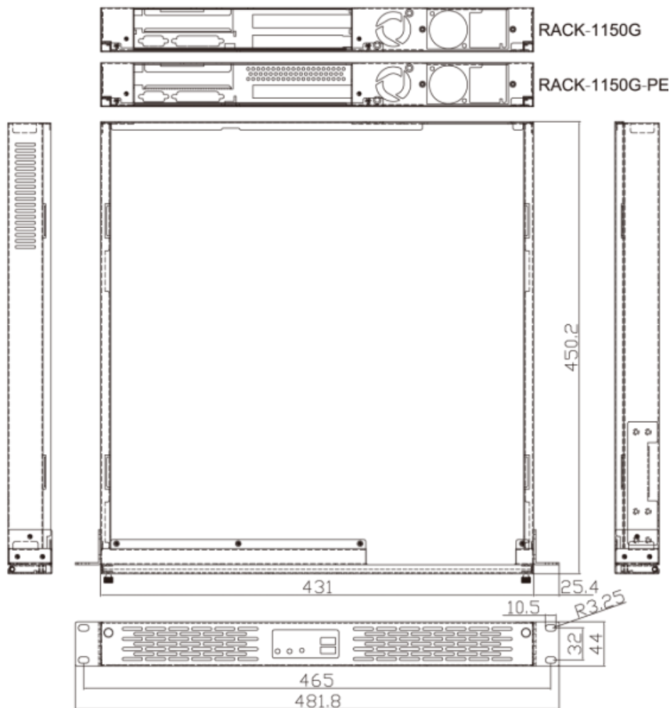
RACK-1150G/1150G-PE Gehäuse bemaßte Zeichnung
